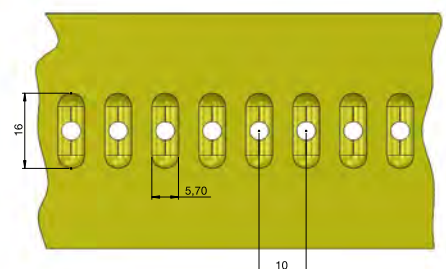
EBPU000399 PU 50T10-920 Aramid NC + PUC060 Yellow 92H x7.5
